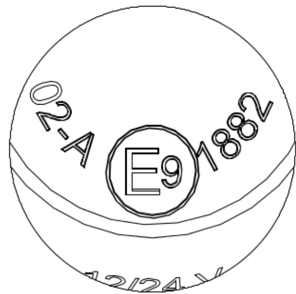
SZCZEGÓŁ A SKALA 5 : 1
